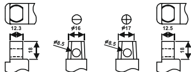
F15 (БОЛТ И ГАЙКА М8)
