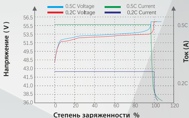
Характеристики заряда при 25°C
