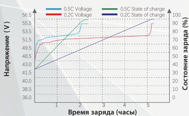
Кривая состояния заряда при 25°C
