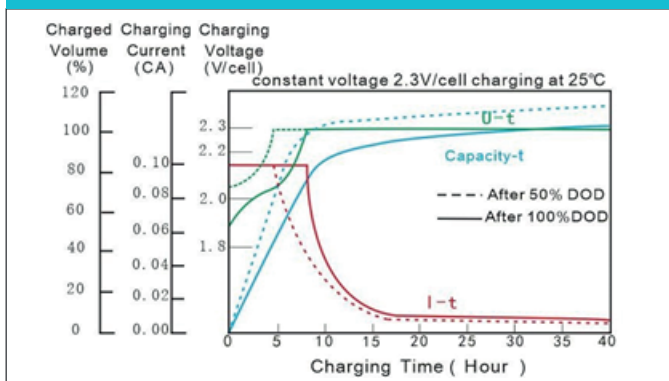
Характеристики заряда
