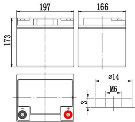
Габаритные размеры, мм
