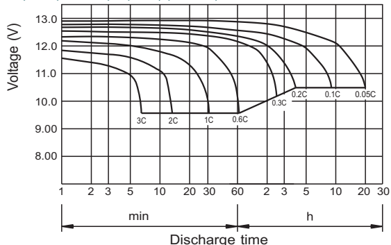
Характеристики разряда (при 25°C)
