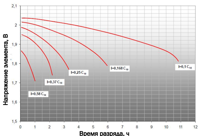
Рис. 1 Стандартные кривые разряда для батарей GEL FIAMM
