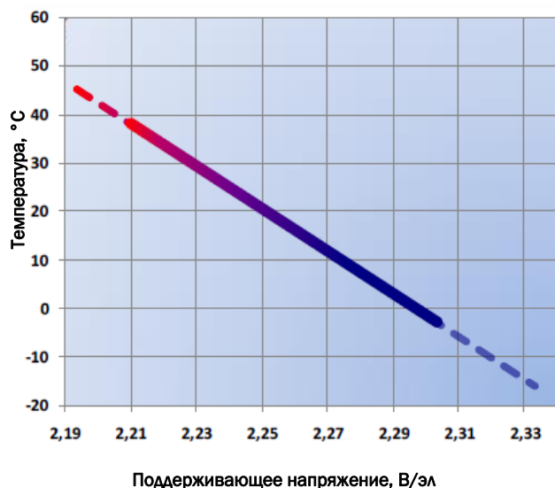
Рис. 6 Рекомендуемое поддерживающее напряжение при различных температурах
