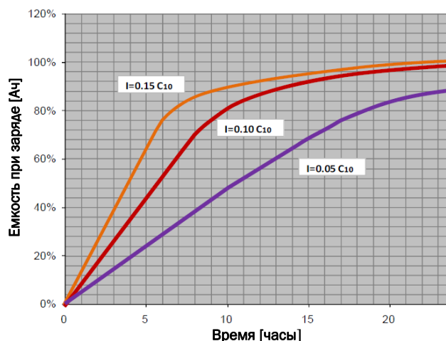
Рис. 7 Кривые заряда при напряжении 2,4 В/эл. с различными пределами тока
