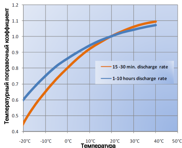
Рис. 3 Поправочный коэффициент для емкости в зависимости от температуры для 10-часового разряда аккумуляторов GEL FIAMM.
