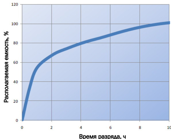
Рис. 2 Зависимость средней фактической емкости от времени разряда для аккумуляторов GEL FIAMM
