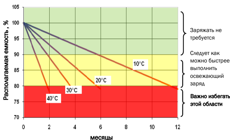
Рис. 8 Время хранения в зависимости от температуры воздуха
