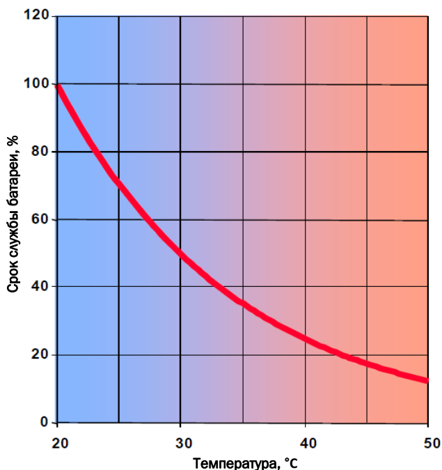
Рис. 4 Ожидаемый срок службы в зависимости от рабочей температуры
