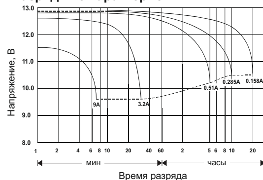
Разрядные характеристики
